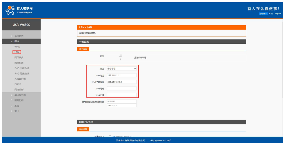
图 9 LAN 设置页面
