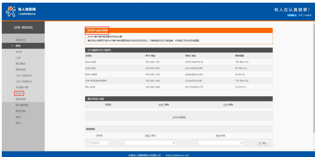
图 19 DHCP 设置页面
