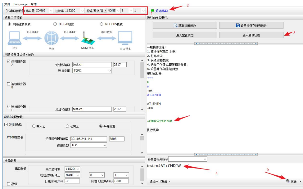
图 78 设置软件示意图
