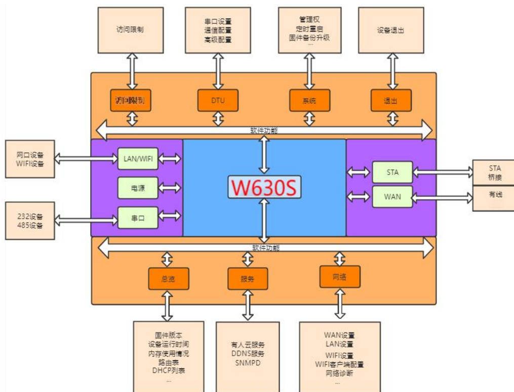
图 3 标准版产品框架图
