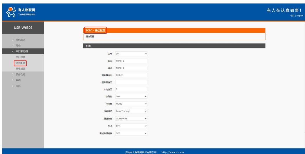
图 25 TCPC 配置界面
