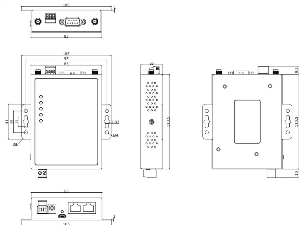
图 1 USR-W630s 尺寸图
