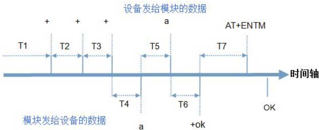
图 77 切换指令模式时序
