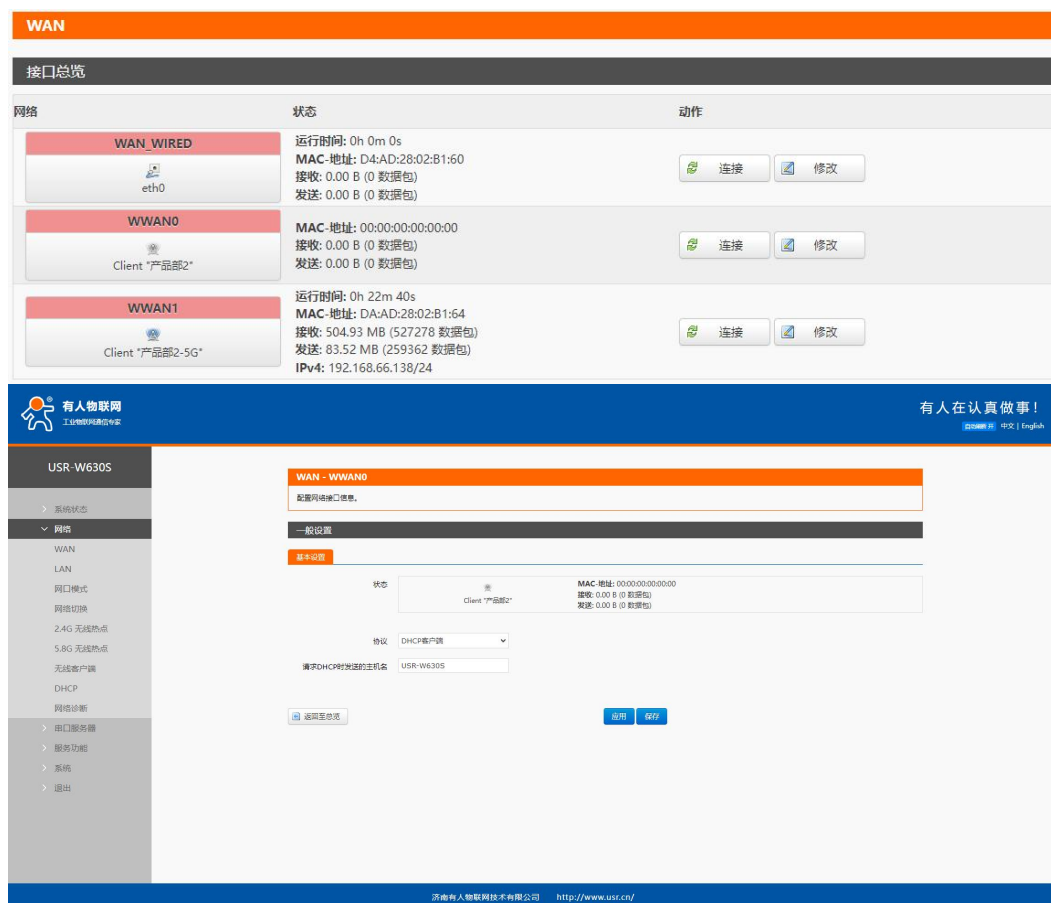
图 4 WAN 口设置页面
