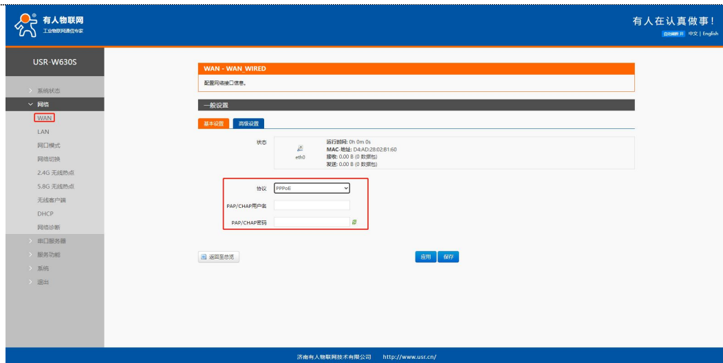
图 7 WAN 口设置-PPPoE
